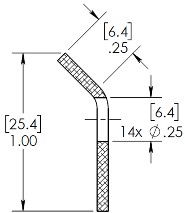
SECTION D-D
